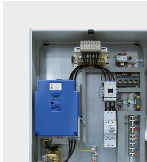
Standard oder kundenspezifisch – Leistungsteile von AERZEN sorgen für den perfekten Motorstart
