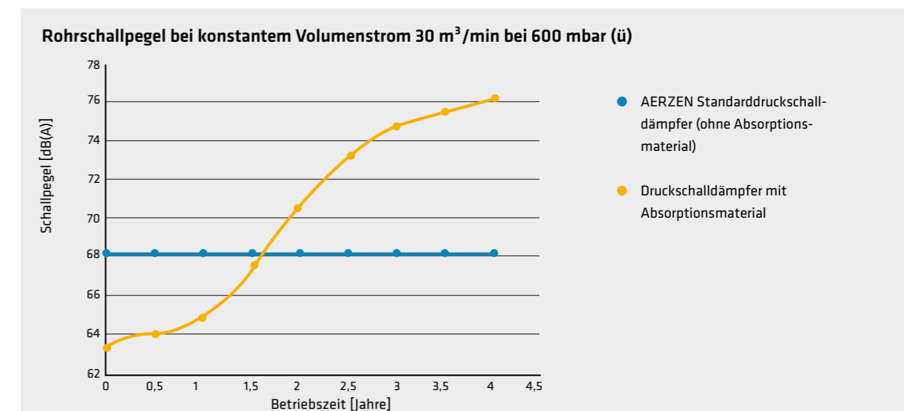
Bild 8: Schallentwicklung durch Verschleiß des Absorptionsmittels im Druckschalldämpfer
